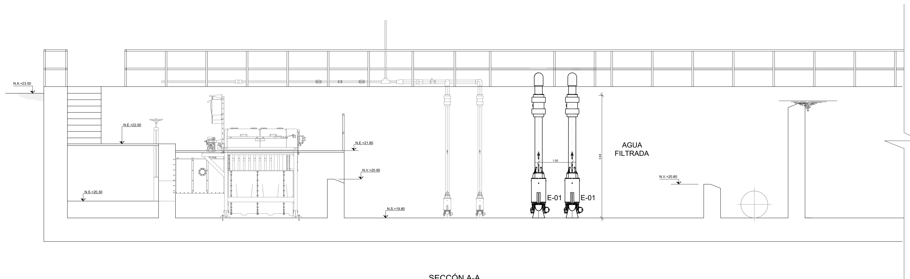
SECCIÓN A-A ESCALA: 1/50
